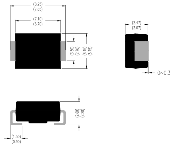
DO-214AB (SMC)
